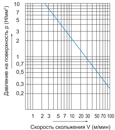
Рис.1 Значение рV
