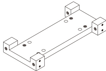
Рис.3 Установка основания и концевых выключателей
