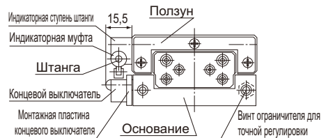
Рис.3 Установка основания и концевых выключателей
