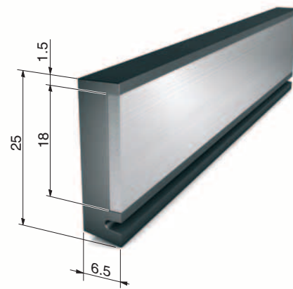
■ Way wiper BA 65-25
