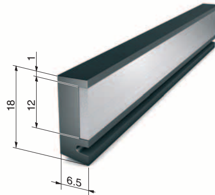
■ Way wiper BA 65-18
