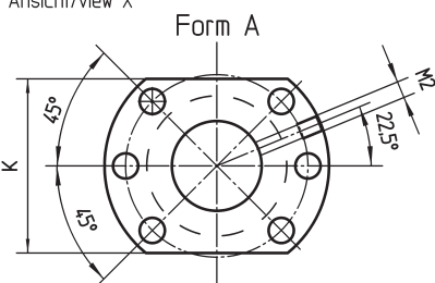
Ansicht/view X
